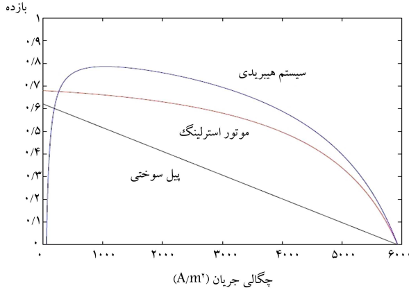
شکل ۵. بازده به چگالی جریان سیستم هیبریدی و اجزای آن.
