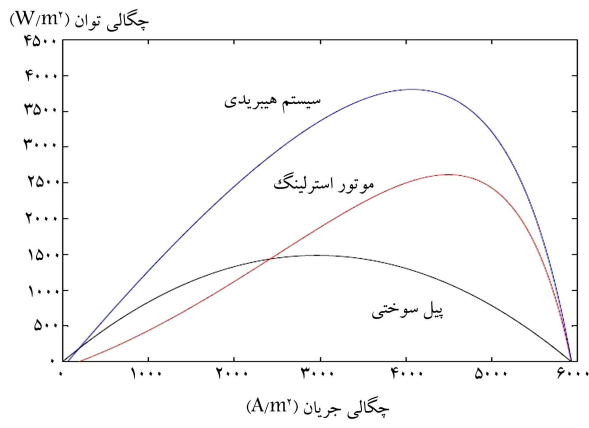
شکل ۶. چگالی توان به چگالی جریان سیستم هیبریدی و اجزای آن.
