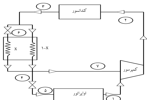
شکل ۳. شماتیک سیکل تبرید با صرفه‌جویی کننده.
