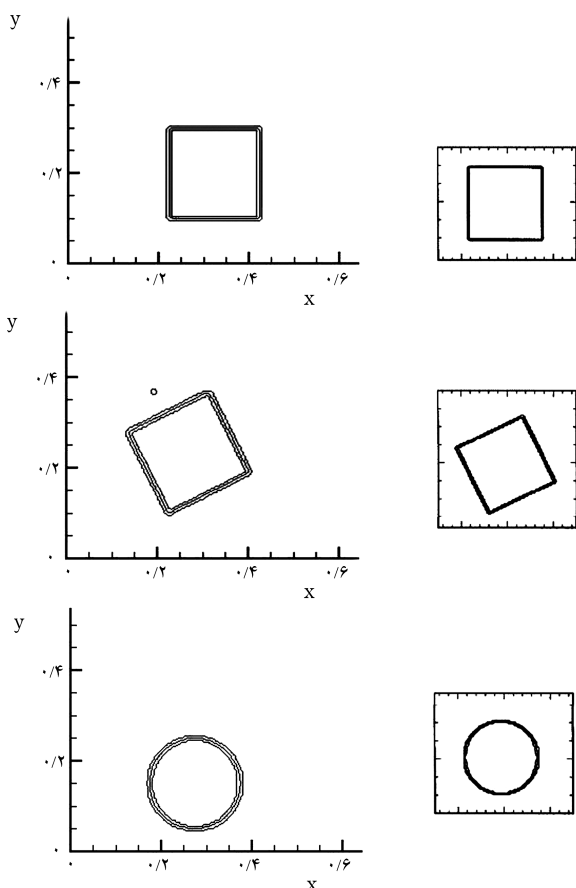
شکل ۷. جابه‌جایی سه ناحیه در میدان سرعت ( u=۱, v=۰ )، نتایج روش VOF-SLIC کار حاضر (ستون سمت چپ)، نتایج روش VOF-SLIC [۱۹] (ستون سمت راست).
