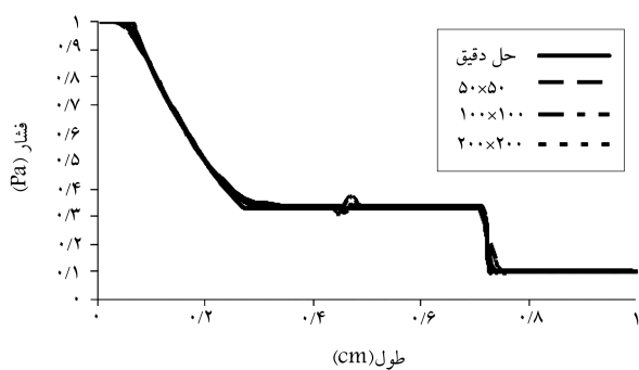
الف) توزیع فشار در طول لوله،
