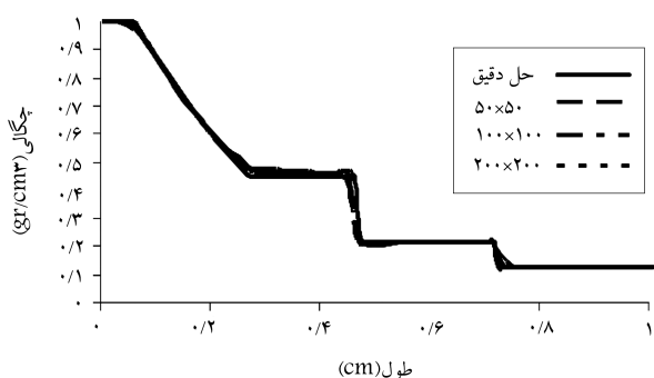
ب) توزیع چگالی در طول لوله.
