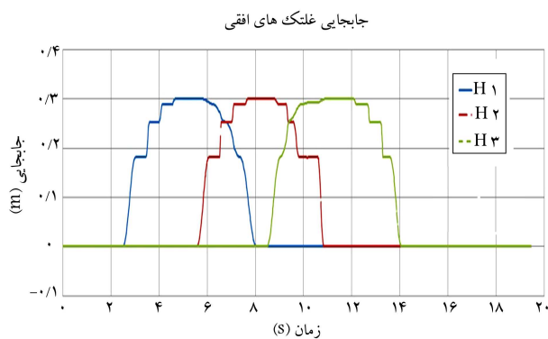
شکل ۸. نمایش جابه‌جایی غلتک‌های افقی برای عبور ربات از گوی اخطار.
