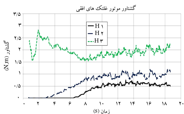
الف) گشتاور غلتک های افقی (H)؛
