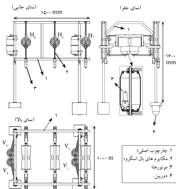
شکل ۲. نمایشی جلو، جانبی و بالای ربات.
