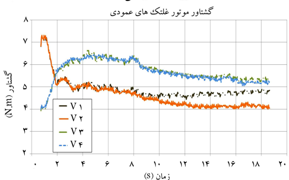
ب) گشتاور غلتک های عمودی (V).
