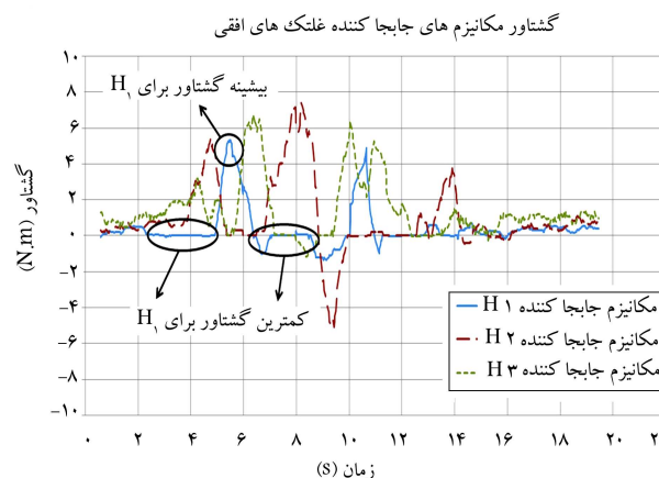
شکل ۹. نمایش گشتاور مورد نیاز غلتک های افقی ربات هنگام عبور ربات از گوی اختار.
