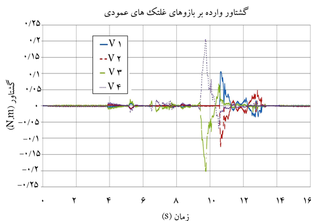
شکل ۱۱. نمایش گشتاور مورد نیاز غلتک های عمودی هنگام عبور ربات از گوی اختار.
