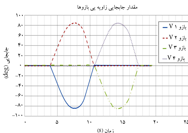
شکل ۱۰. نمایش جابه جایی زاویه ی غلتک های عمودی هنگام عبور از گوی اختار.
