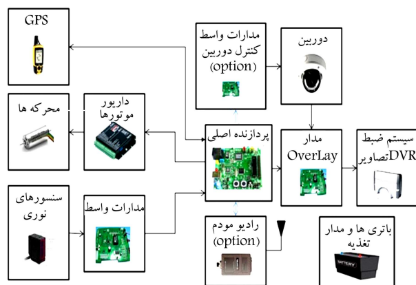
شکل ۴. ارتباط بین سیستم کنترل و تجهیزات جانبی ربات.
