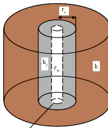
شکل ۱. مخزن همگن با آسیب‌سازندی.
