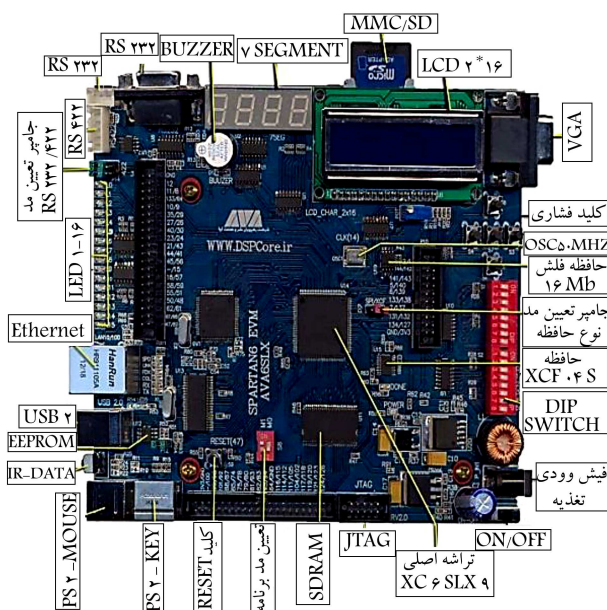
شکل ۱. بورد FPGA مورد استفاده.
