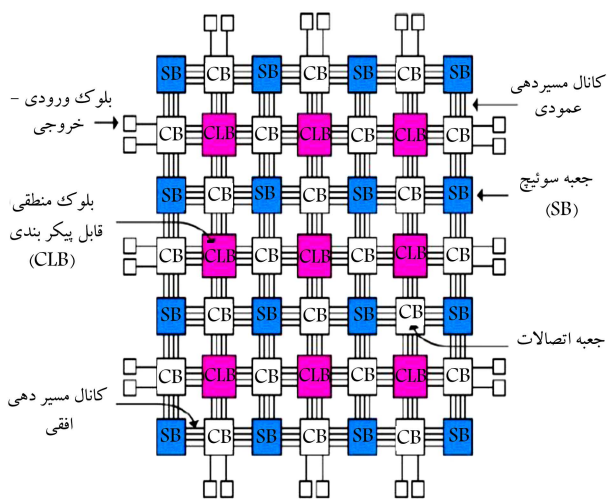
شکل ۲. ساختار داخلی FPGA.
