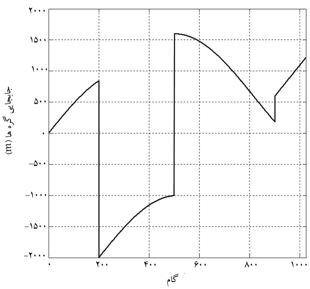
شکل ۱۱. منحنی حرکت گره ۵ در حالت پیاده‌سازی سخت‌افزاری بدون استفاده از رجیستر.
