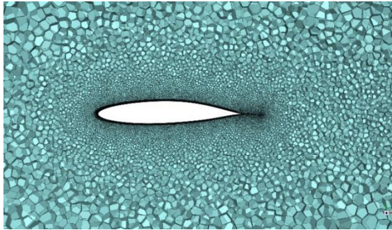
شکل ۹: شبکه محاسباتی اطراف ایرفویل.
