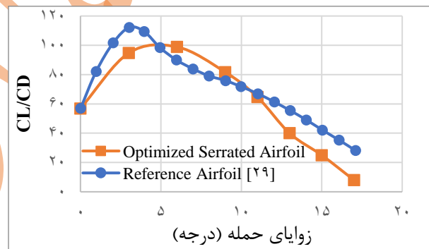
شکل ۱۷: مقایسه نتایج نسبت ضریب برآ به پسا برای ایرفویل دنداندار بهینه‌شده با ایرفویل معیار.
