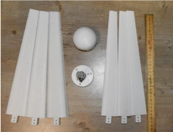
شکل ۶: پره‌های معیار و بهینه تولیدشده توسط پرینت سه بعدی.
