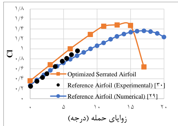
شکل ۱۶: مقایسه نتایج ضریب برآ برای ایرفویل دنداندار بهینه‌شده با ایرفویل معیار.
