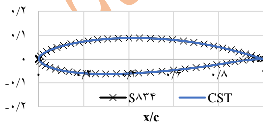
شکل ۱: مقایسه بین S834 واقعی و نمایش CST.
