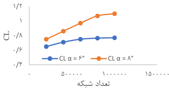
شکل ۱۱: منحنی استقلال از شبکه.
