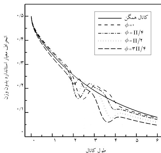
شکل ۵. میزان غلظت متوسط و انحراف معیار در طول چند ریزمجرا با دیواره‌ی ناهمگن ( Sc=50 ).
