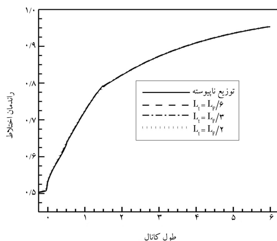
شکل ۱۵. میزان اختلاط در طول ریزمجرای برای پروفیل‌های منقطع و پیوسته از سرعت لغزشی در دیواره.
