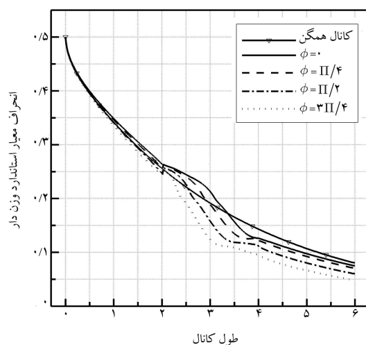
شکل ۶. میزان غلظت متوسط و انحراف معیار وزن‌دار با تابع وزنی سرعت در طول چند ریزمجرا با دیواره‌ی ناهمگن ( Sc=50 ).
