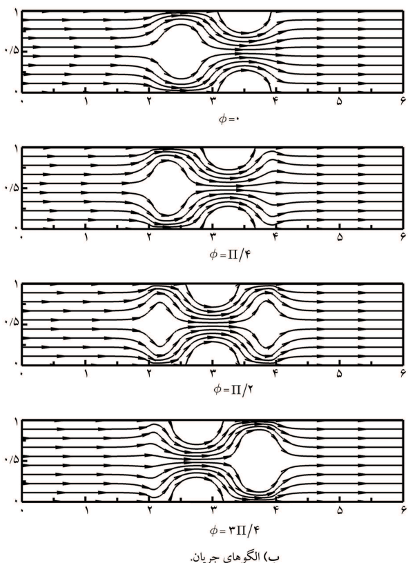
شکل ۴. جریان مورد مطالعه برای ارزیابی معیارهای اختلاط درون ریزمجرای ناهمگن.
