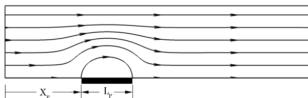
شکل ۳. ساده‌ترین نحوه‌ی ایجاد ریزمجرای ناهمگن و خطوط جریان مربوط به آن.
